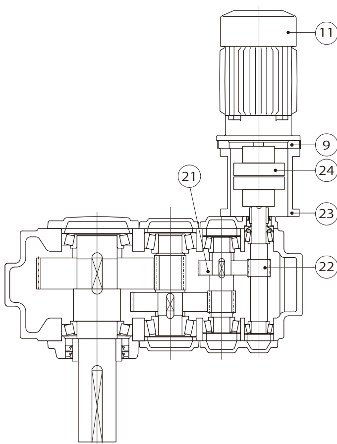
図11-4 ドライブユニット平行軸横形3段
